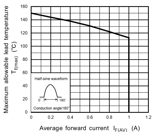
Fig. 10.5 T_{t(max)} - I_{F(AV)}
