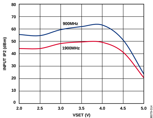
Figure 14. Input IP2 vs. VSET
